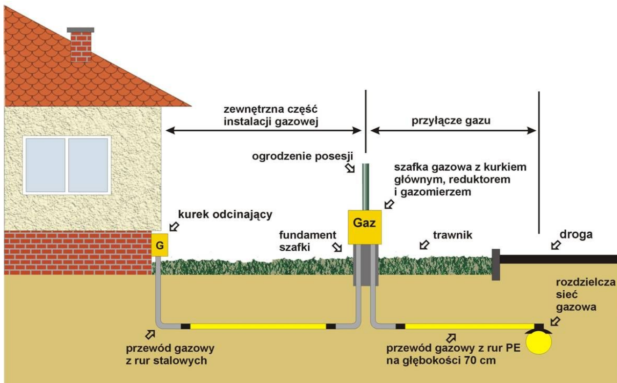
Schemat przykładowego przyłącza.
